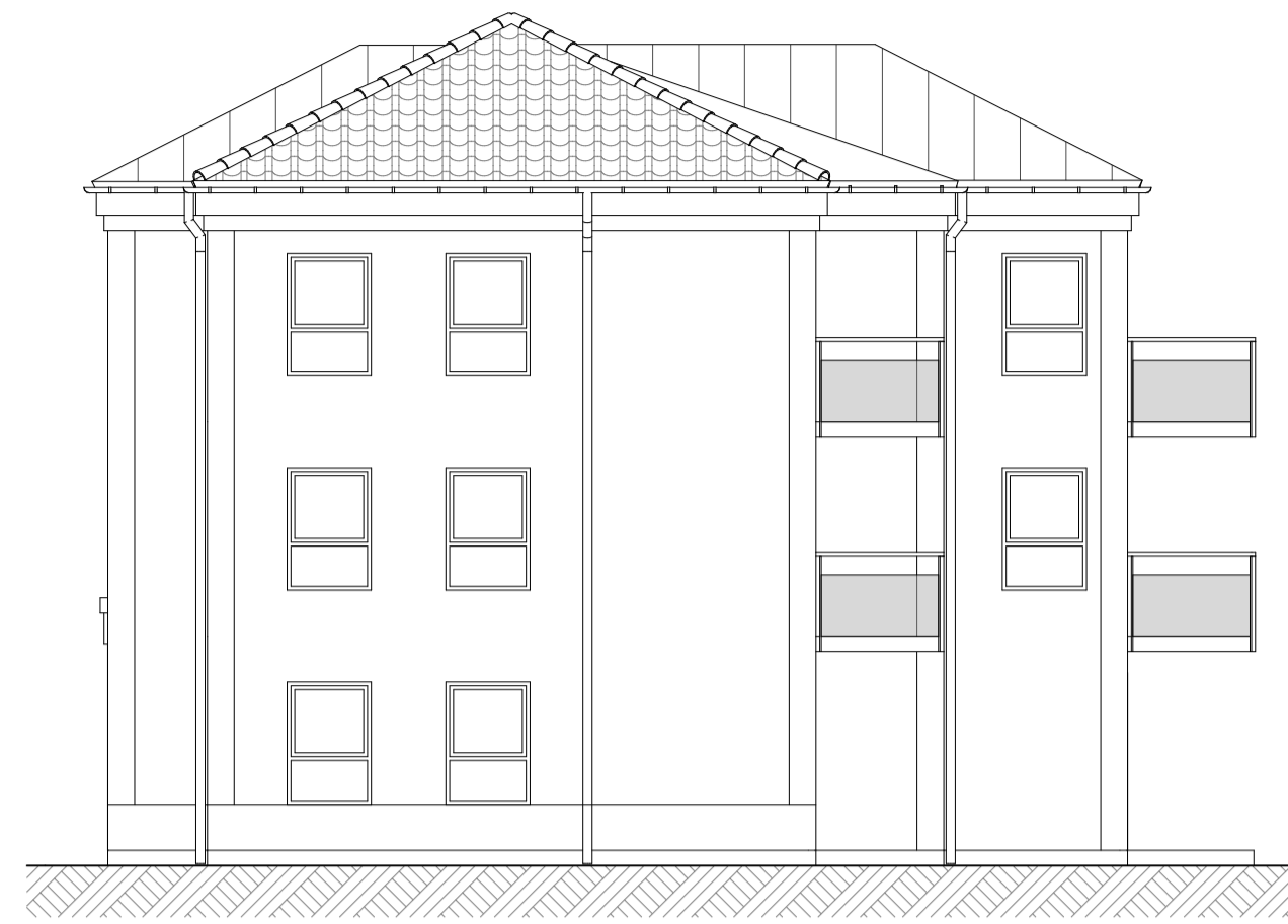
Fasad mot nordost 1:100
