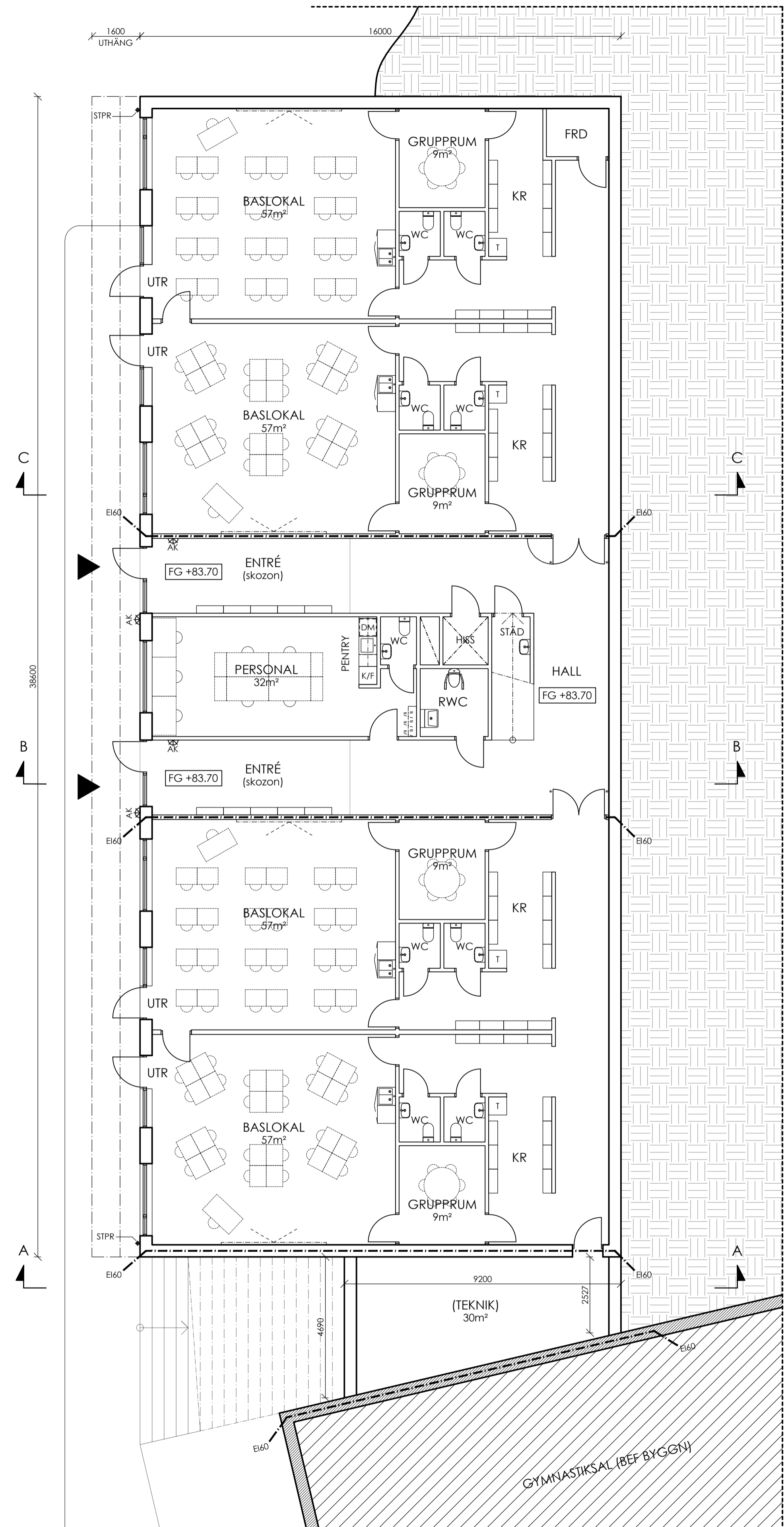
PLAN 09 (SOUTERRÄNG) SKALA 1:100 (A1)
